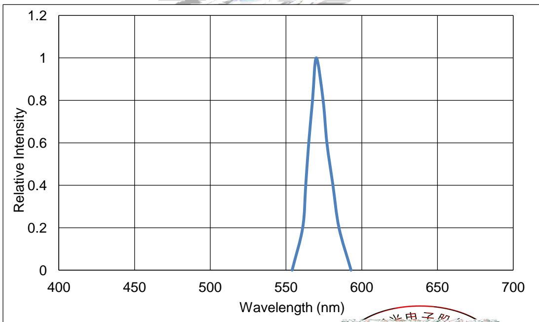
Fig 1-11 Relative Intensity Vs Wavelength (Ta=25°C) 相对强度与主波长关系曲线
