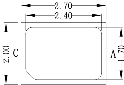
正面视图
