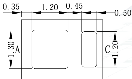
背面视图
